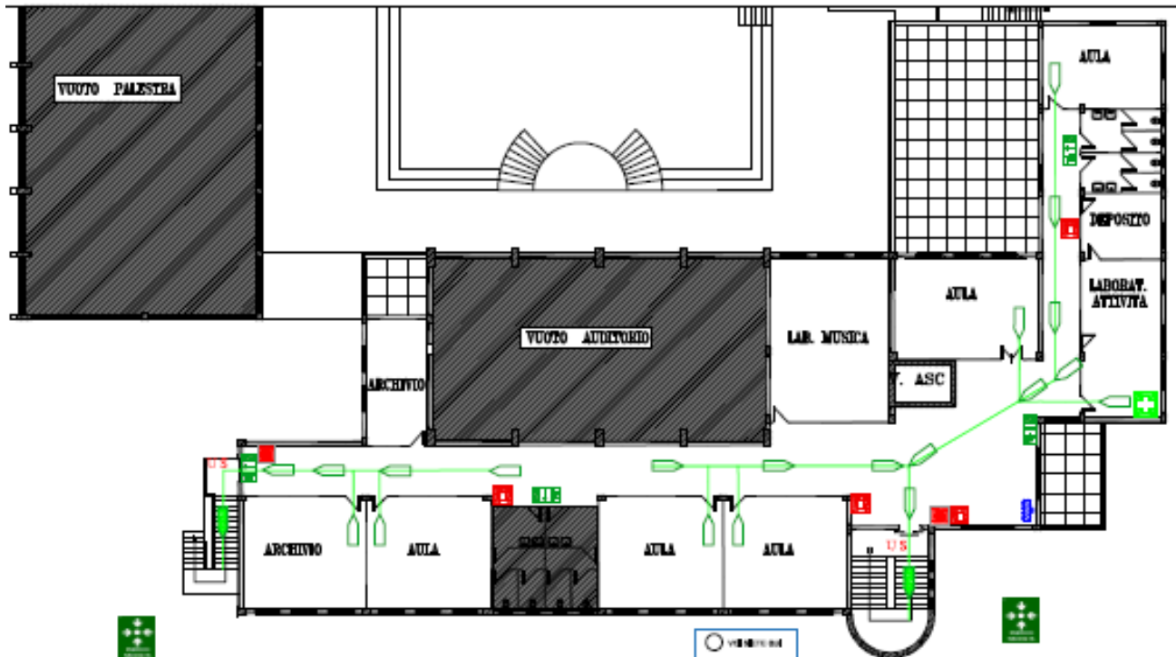
FRASCINETO - VIA F.LL. CERV. - PIANO DI EVACUAZIONE - PIANO PRIMO
